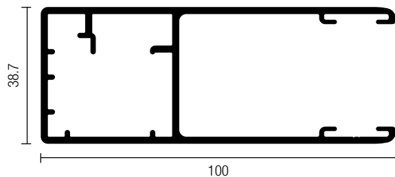
Perfil Portão
